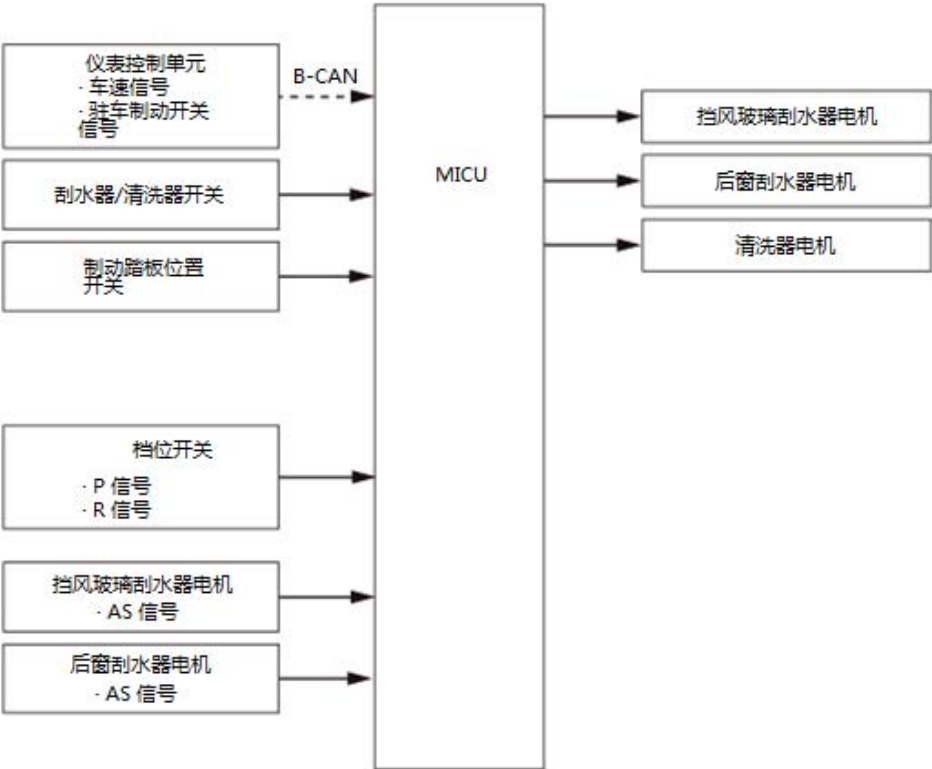
刮水器/清洗器系统说明 - 系统图
